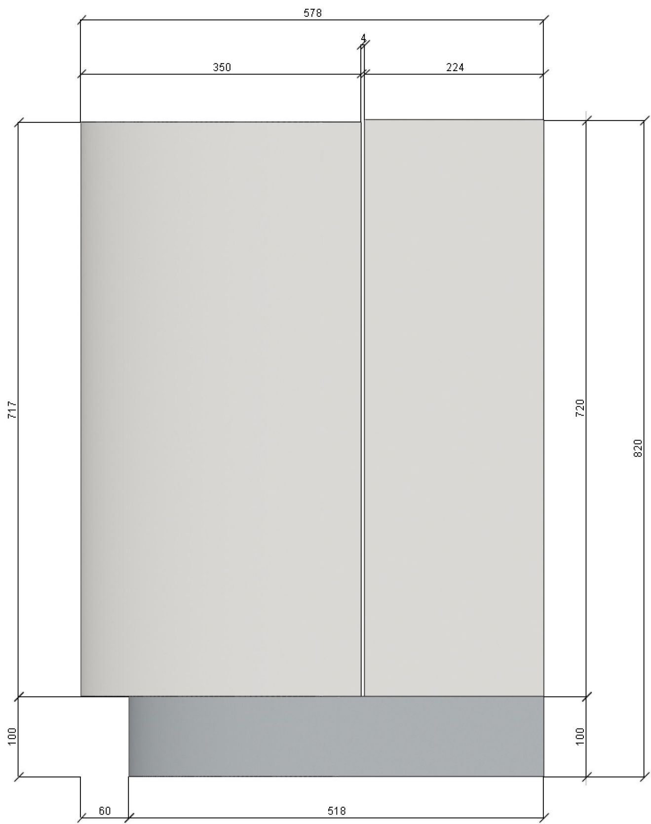
Przekrój boczny przez szafkę giętą dolną
